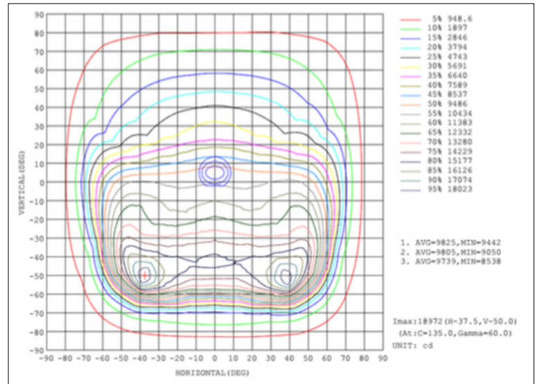
LL-ALL-295-50-UNV-T3-BZ
