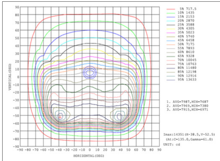
LL-ALL-235-50-UNV-T3-BZ
