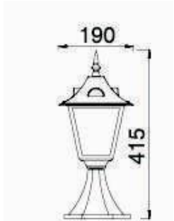
OGLD04C
