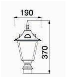
OGLD04
