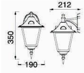
OGLD04B
